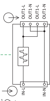
DGTM104 1 x 4 A TE dimmer module
