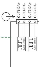
DGBM200 2 CH Driver module
